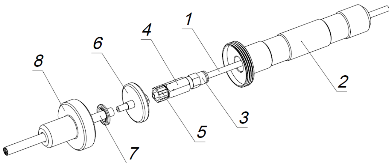
Рис. 1.3. Схема пробоотборника
