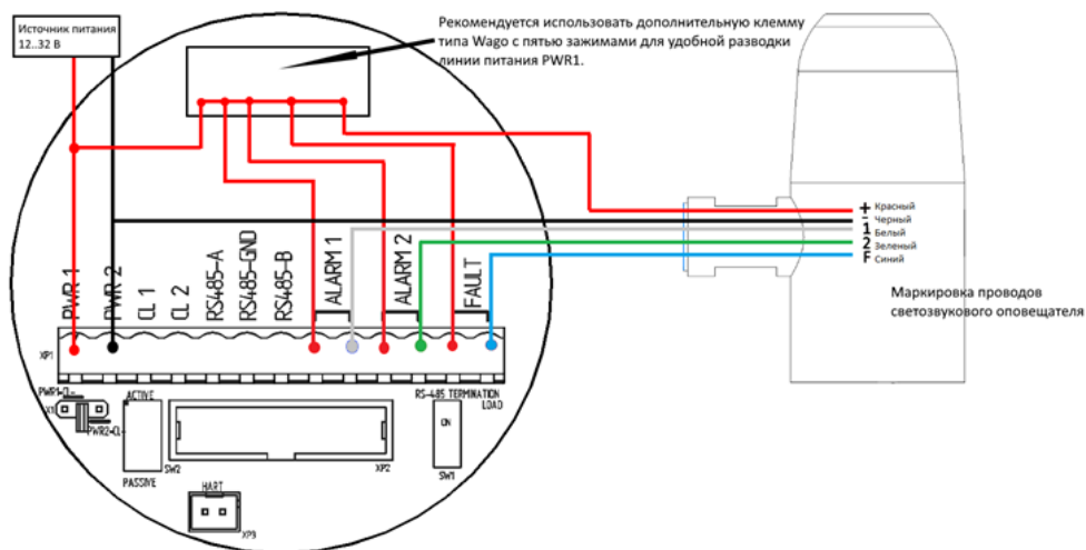
Рисунок 22 – Схема подключения светозвукового сигнализатора ЭМИ-СЗ к ИГМ-12М, изготовленным до апреля 2023г.
