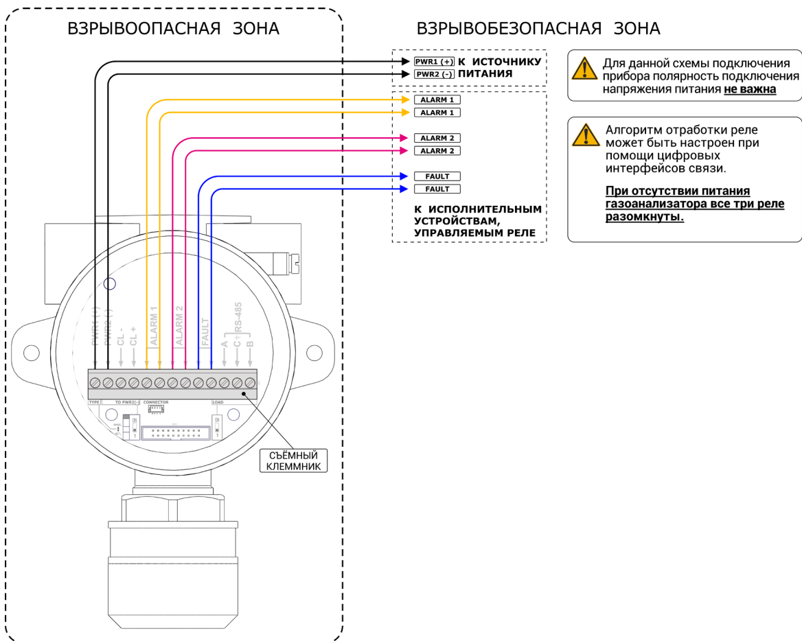
Рисунок И.8 – Подключение внешних исполнительных устройств к реле газоанализатора
