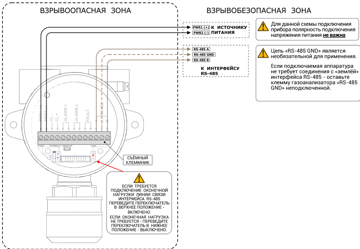
Рисунок И.7 – Подключение по интерфейсу RS-485
