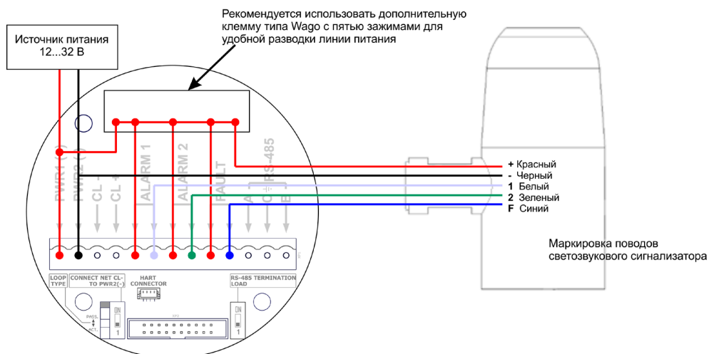
Рисунок 23 – Схема подключения светозвукового сигнализатора ЭМИ-СЗ к ИГМ-12М, изготовленным с апреля 2023г.
