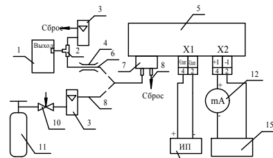
в) для газоанализаторов ДАХ-М-05X-Н 2 -S-40, ДАХ-М-05X-SO 2 -20, ДАХ-М-05X-Cl 2 -25, ДАХ-М-05X-Cl 2 -50, ДАХ-М-05X-NO 2 -10, ДАХ-М-05X-N 2 O 2 -20, ДАХ-М-05X-HCl-30, ДАХ-М-05X-RSH-5
