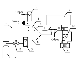
б) для газоанализаторов ДАХ-М-04-Н 2 -S-40, ДАХ-М-04-SO 2 -20, ДАХ-М-04-Cl 2 -25, ДАХ-М-04-Cl 2 -50, ДАХ-М-04-NO 2 -10, ДАХ-М-04-N 2 O 2 -20, ДАХ-М-04-HCl-30, ДАХ-М-04-RSH-5
