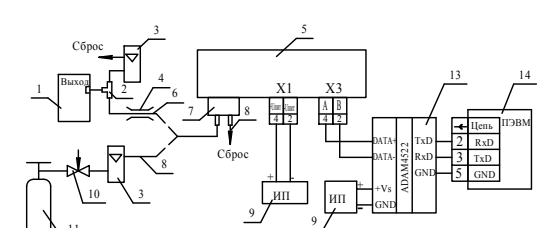
д) для газоанализаторов ДАХ-М-06-Н 2 -S-40, ДАХ-М-06-SO 2 -20, ДАХ-М-06-Cl 2 -25, ДАХ-М-06-Cl 2 -50, ДАХ-М-06-NO 2 -10, ДАХ-М-06-N 2 O 2 -20, ДАХ-М-06-HCl-30, ДАХ-М-06-RSH-5
