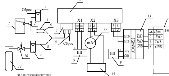
з) для газоанализаторов ДАХ-М-06TRX-Н 2 -S-40, ДАХ-М-06TRX-RSH-5, ДАХ-М-06TRX-SO 2 -20, ДАХ-М-06TRX-Cl 2 -25, ДАХ-М-06TRX-Cl 2 -50, ДАХ-М-06TRX-NO 2 -10, ДАХ-М-06TRX-N 2 O 2 -20, ДАХ-М-06TRX-HCl-30, ДАХ-М-06TRXH-Н 2 -S-40, ДАХ-М-06TRXH-RSH-5, ДАХ-М-06TRXH-SO 2 -20, ДАХ-М-06TRXH-Cl 2 -25, ДАХ-М-06TRXH-Cl 2 -50, ДАХ-М-06TRXH-NO 2 -10, ДАХ-М-06TRXH-N 2 O 2 -20, ДАХ-М-06TRXH-HCl-30
