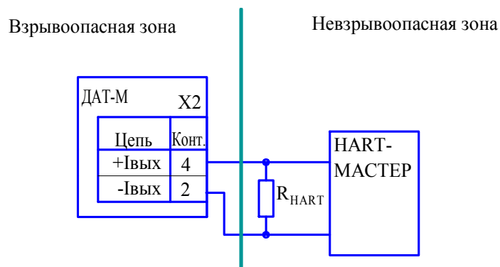
а) подключение HART-мастера при отсутствии подключения выходного сигнала постоянного тока
