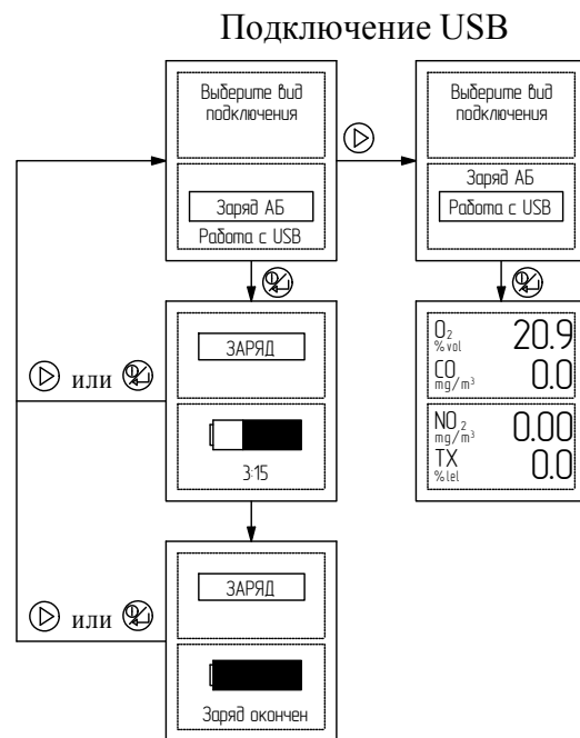
Рисунок Д.4
