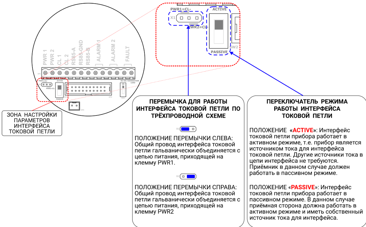
Рисунок 22 – Настройка параметров интерфейса токовой петли для ИГМ-11, изготовленных до апреля 2023г.
