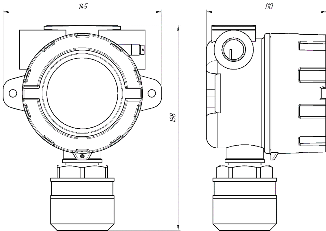
Рисунок 5 – Габаритные размеры ИГМ-11 (корпус тип 1)
