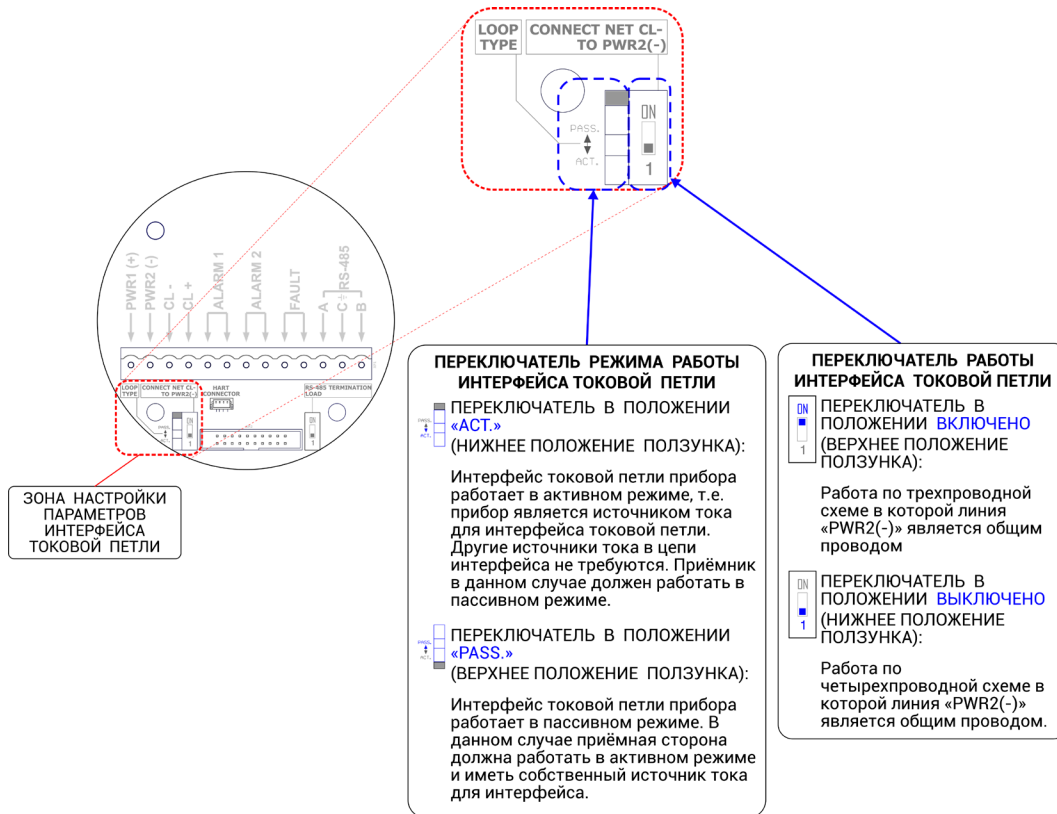
Рисунок 23 – Настройка параметров интерфейса токовой петли для ИГМ-11, изготовленных с апреля 2023г.
