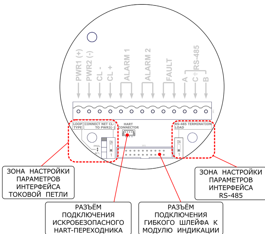
Рисунок 13 – Расположение и функциональное назначение переключателей настройки параметров работы интерфейсов ИГМ-11, изготовленных с апреля 2023г.
