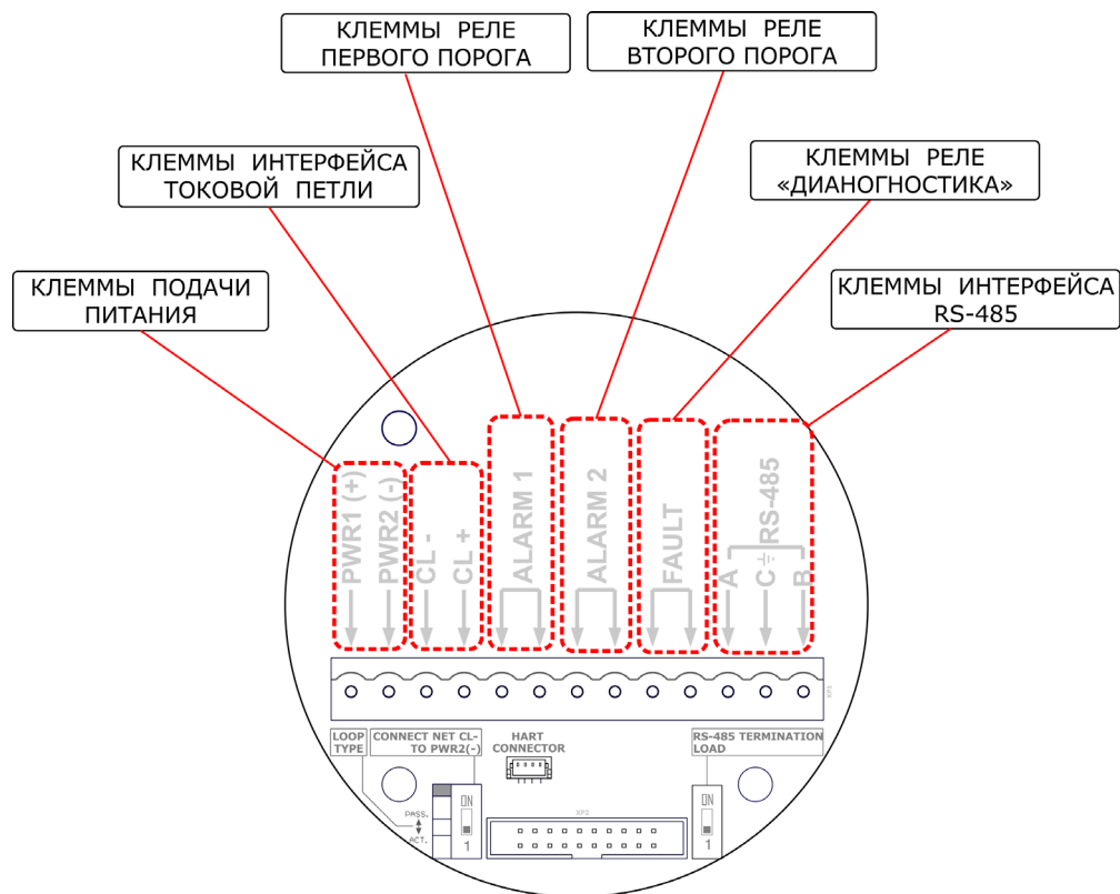
Рисунок 12 – Функциональное назначение клемм подключения внешних электрических цепей ИГМ-11, изготовленных с апреля 2023г.
