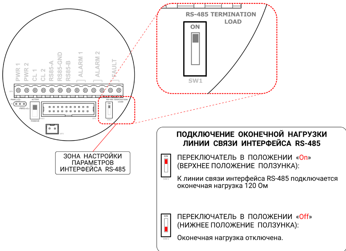
Рисунок 24 – Подключение оконечной нагрузки линии связи интерфейса RS-485 для ИГМ-11, изготовленных до апреля 2023г
