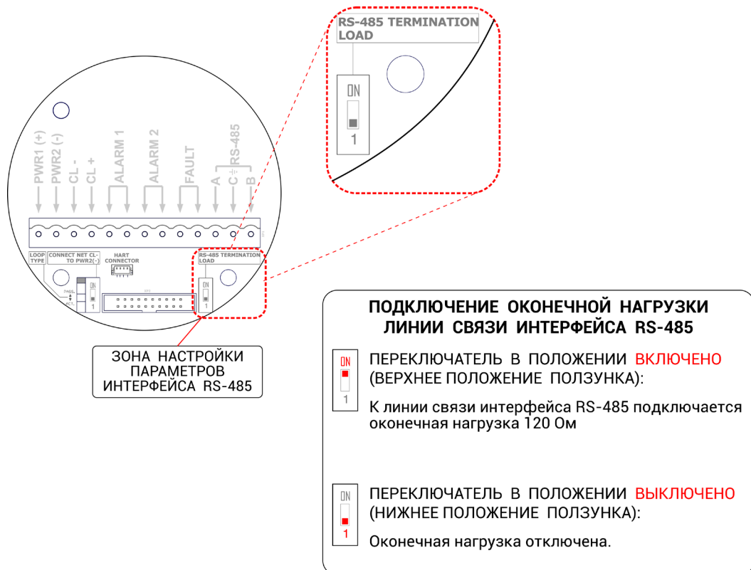
Рисунок 25 – Подключение оконечной нагрузки линии связи интерфейса RS-485 для ИГМ-11, изготовленных с апреля 2023г.
